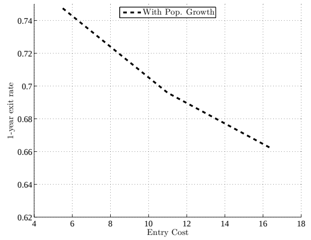
(d) Conditional exit rate
